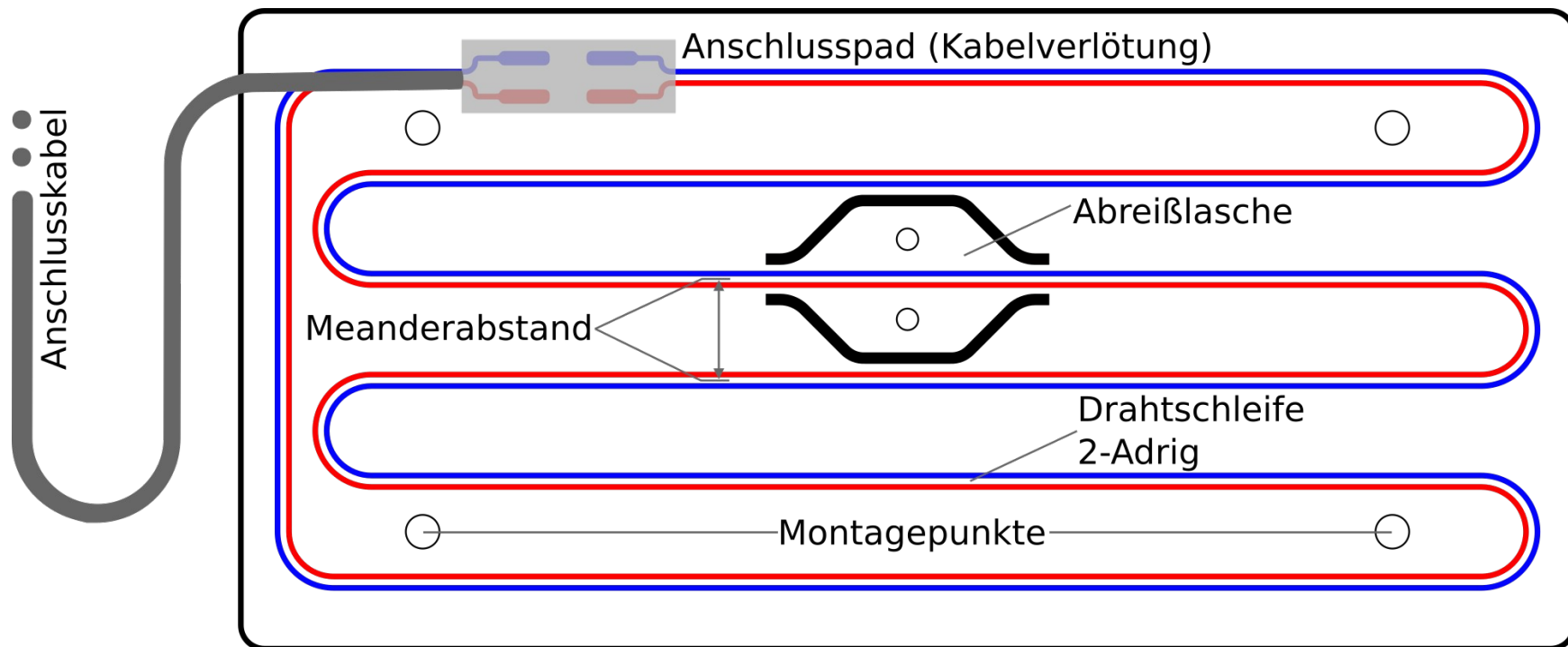
(Abbildung 1) - Version mit einfachem Kabelanschluss („SingleWire“)
