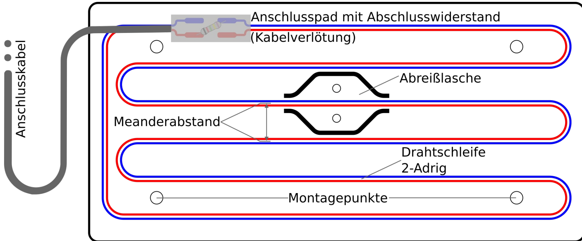
(Abbildung 3) - Version mit einfachem Kabelanschluss und Abschlusswiderstand integriert („SingleWireResistor“)
