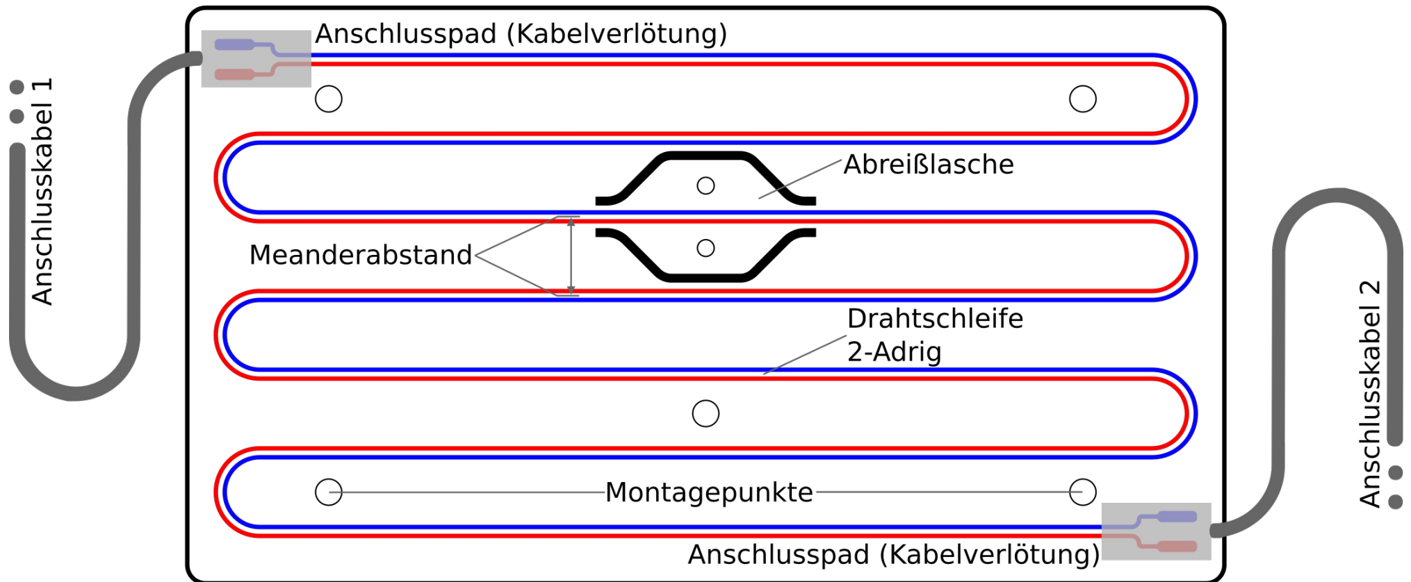
(Abbildung 2) - Version mit doppeltem Kabelanschluss – diagonal („DoubleWire“)
